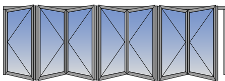
Με μονό αριθμό φύλλων στη μία πλευρά
